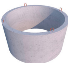
Бетонное кольцо стеновое КС 20-9
